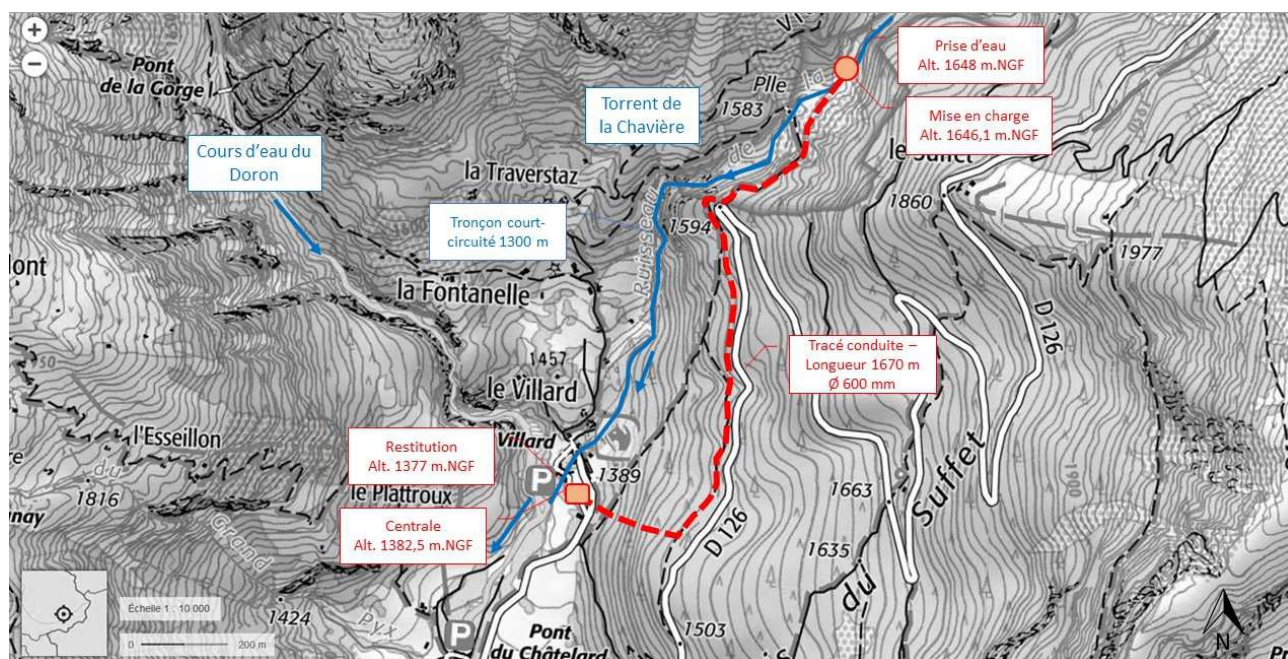
Figure 2: Projet de centrale hydroélectrique – Plan de situation au 1/10 000ème (source: résumé non technique)
