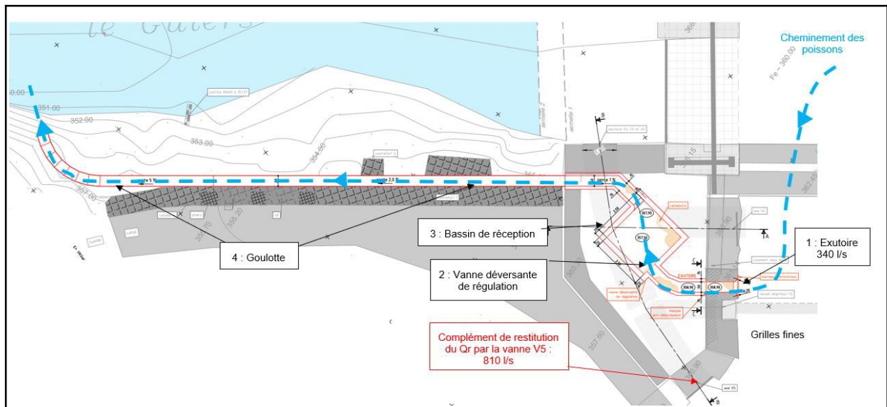
Schéma de principe de du dispositif de dévalaison (vue en plan)
